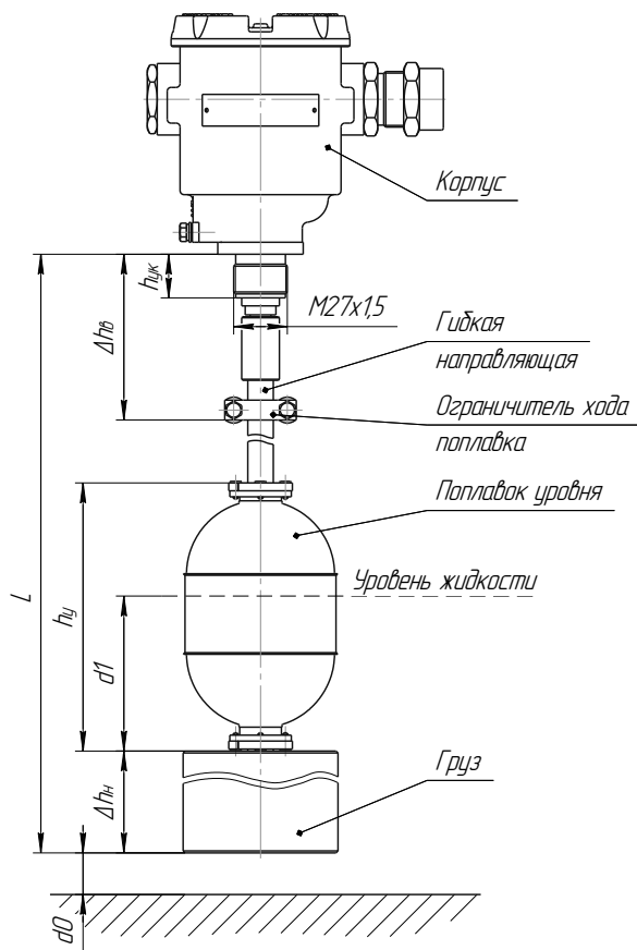
Рисунок 1 – Общий вид уровнемера
