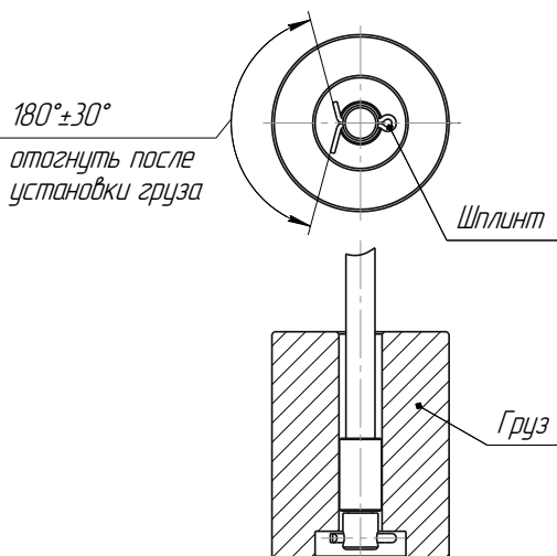
Рисунок 6 – Установка груза
