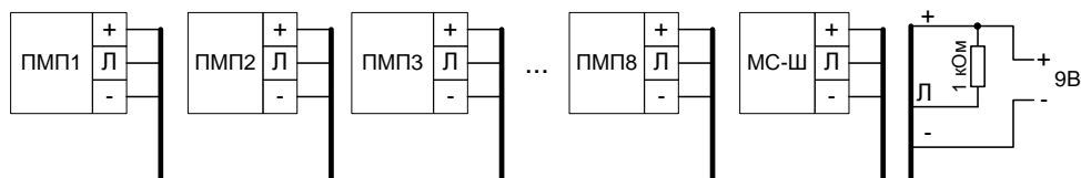
Линия питания-связи системы СЕНС
