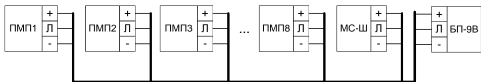
Линия питания-связи системы СЕНС
