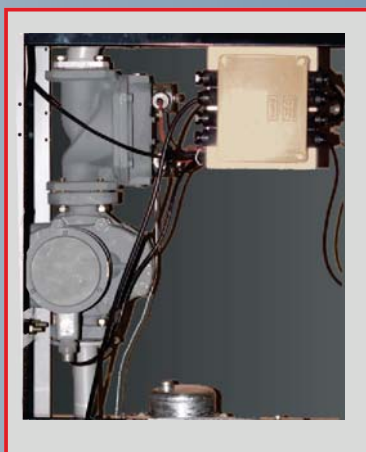
Блок гидравлики с измерителем объема ППО
